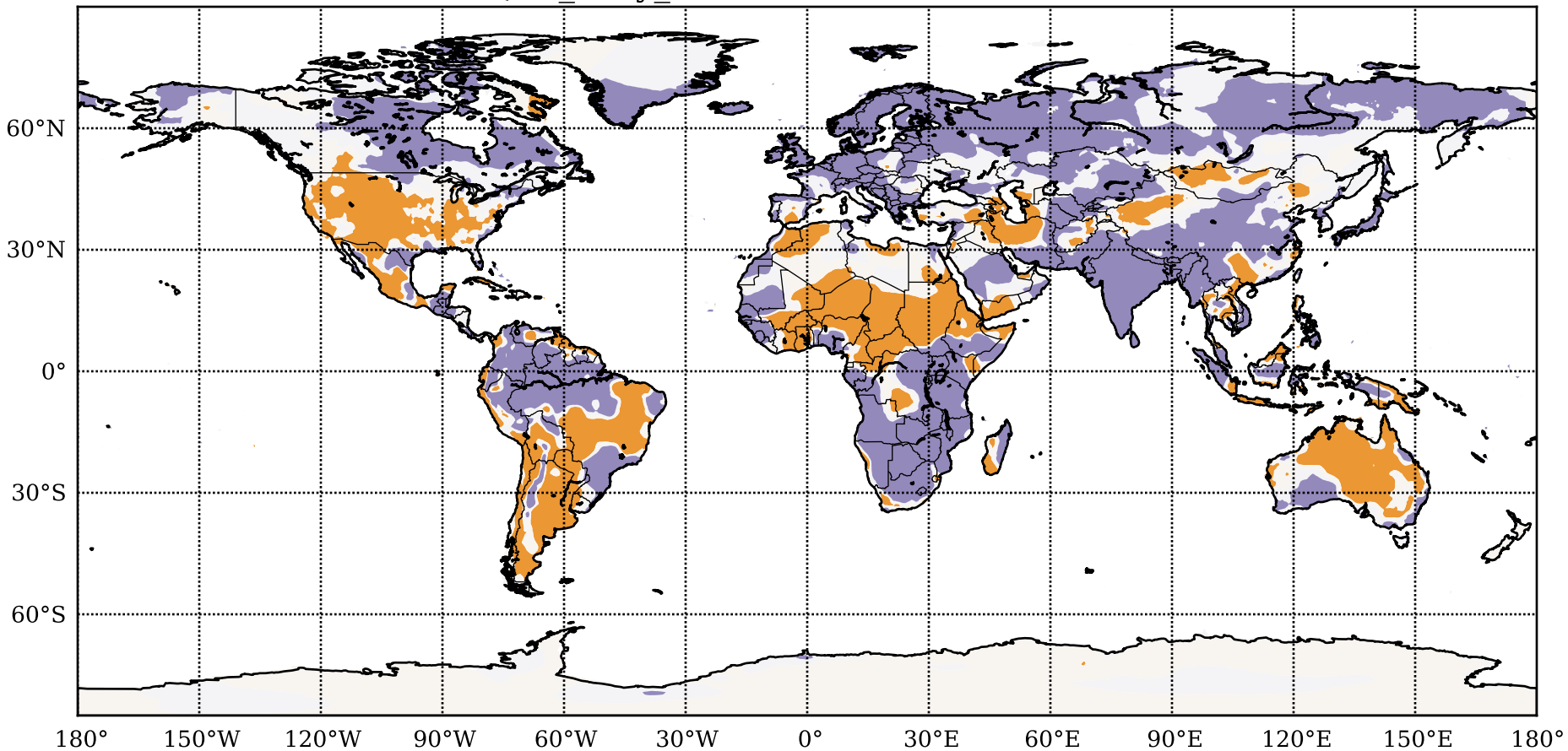
Qair_daily_WFDEI: 1979-2009, TREND
