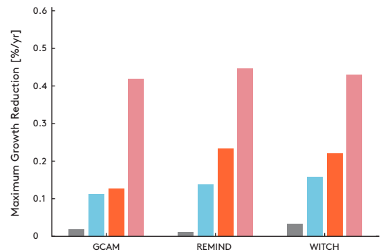
(d) Unused fossil capacities (max 2010–2050)
