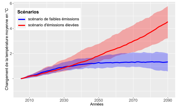
Figure 1 : Évolution des température annuelles moyennes sur 21 années consécutives au Niger.
