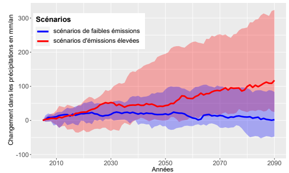
Figure 2 : Évolution des quantités de précipitations annuelles moyennes sur 21 années consécutives au Niger.
