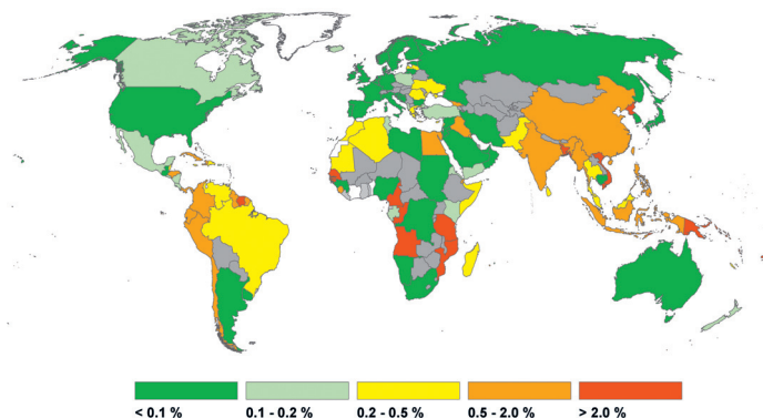
Abb. 2: Zunahme des Bevölkerungsanteils in Regionen, die ohne verstärkten Küstenschutz durch den Meeresspiegelanstieg jährlich überflutet würden (bezogen auf den Zeitraum 2000–2070).
