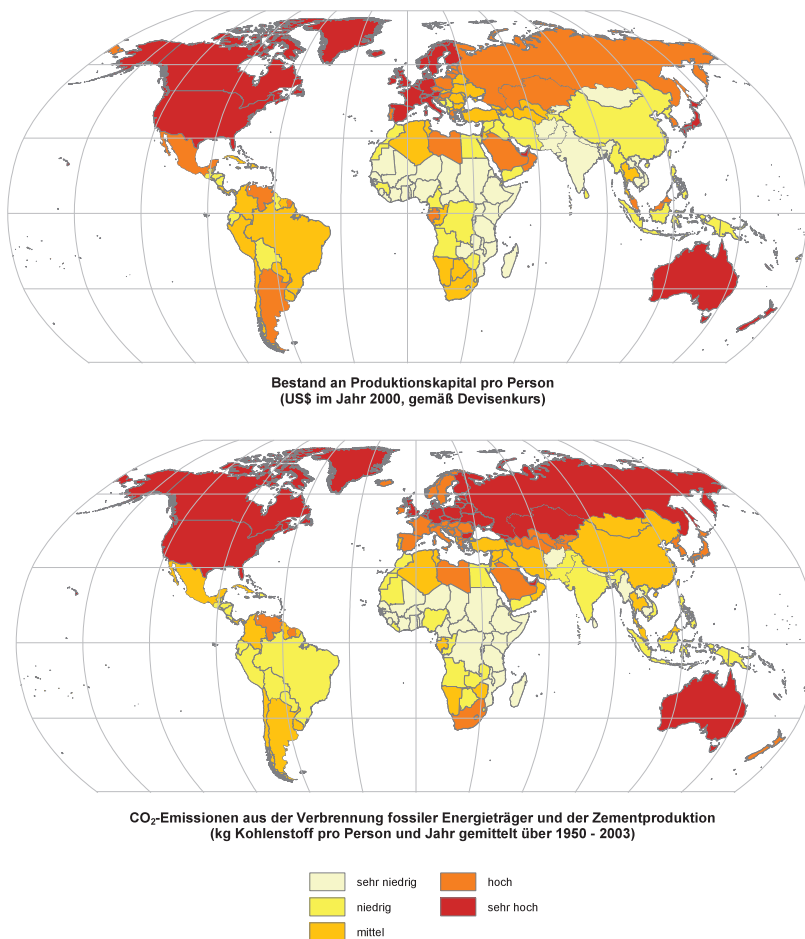
Abb. 3: Verteilung des globalen Vermögens pro Person für das Jahr 2000 und der historischen Emissionen für den Zeitraum von 1950–2003.
