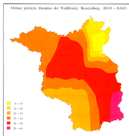
Abb. 5: Mittlere jährliche Zunahme der Waldbrände, Brandenburg, (SG30 - BASZ)
