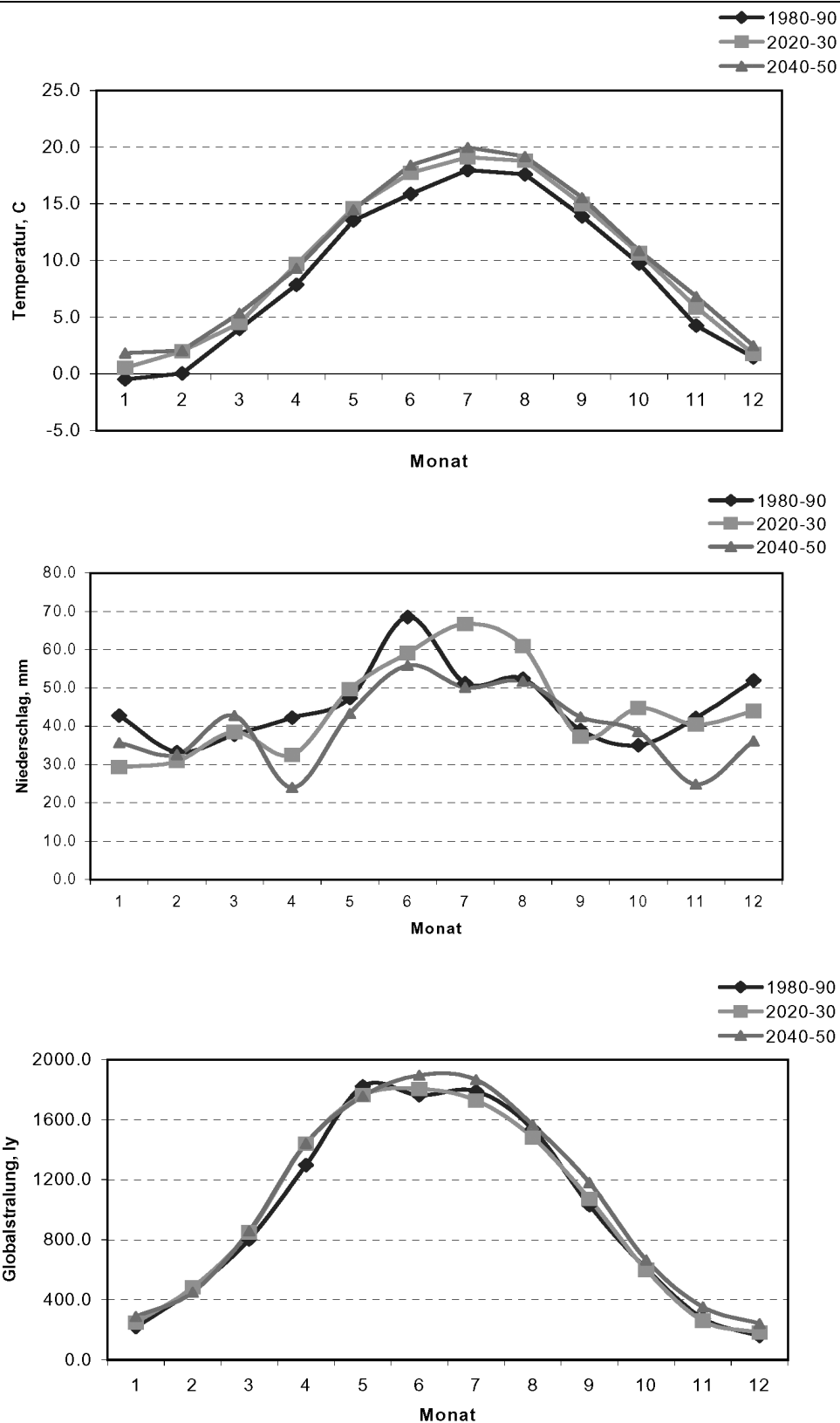
Abb. 33: Klimacharakteristiken für das Referenzklima (1980-1990) und das Klimaszenarium.
