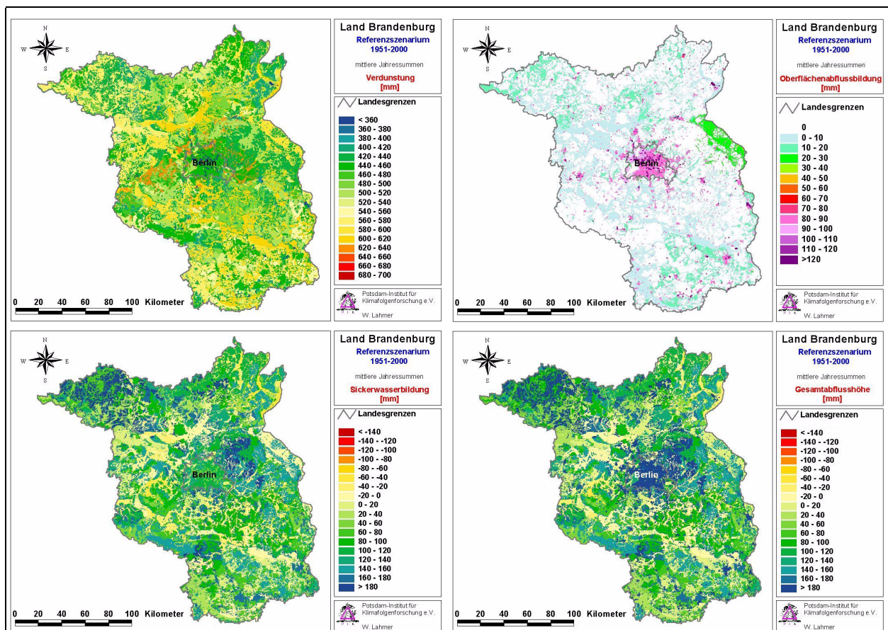
Abb. 18: Flächendarstellungen der für das Land Brandenburg berechneten Verdunstung, Sickerwasserbildung, Oberflächenabflussbildung und Gesamtabflusshöhe für das Referenzszenarium (beobachtetes Klima im Zeitraum 1951-2000).
